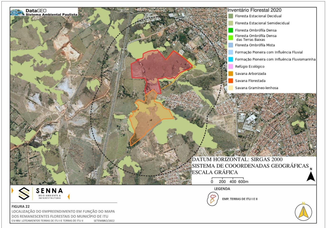
FIGURA 22: Localização da ADA (laranja) em função do mapa dos remanescentes florestais do município de Itu, em detalhe (Instituto Florestal do Estado de São Paulo – adaptado de datageo.ambiente.sp.gov).
