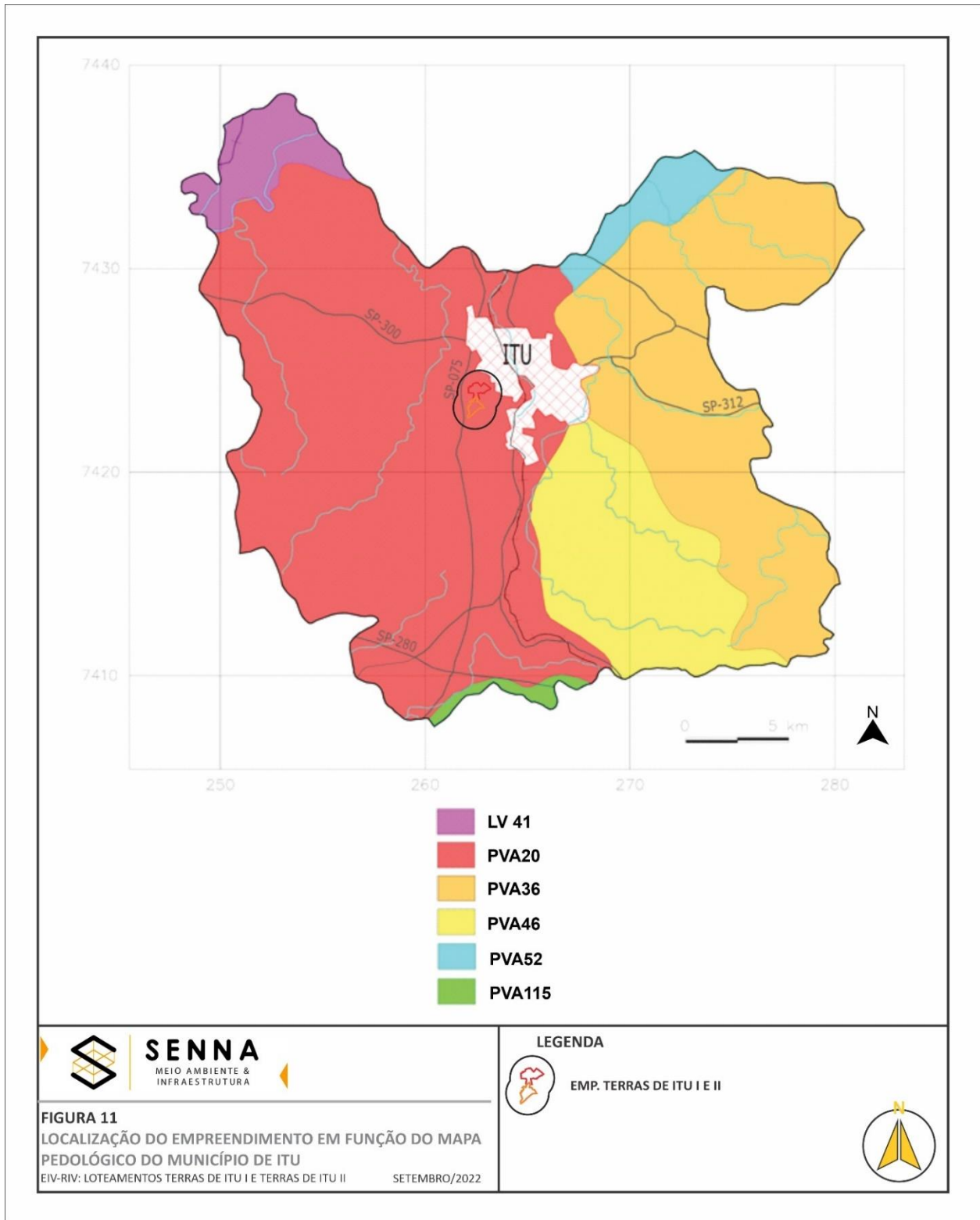
FIGURA 11: Localização da área de estudos, em função do Mapa Pedológico do município de Itu (adaptado de IPT, 1981).
