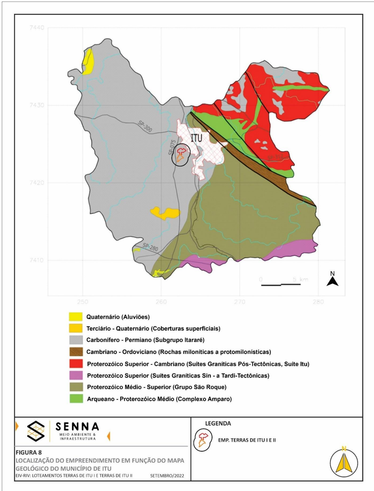
FIGURA 8: Localização da área, em função do mapa geológico do município de Itu (adaptado de IPT, 1981).
