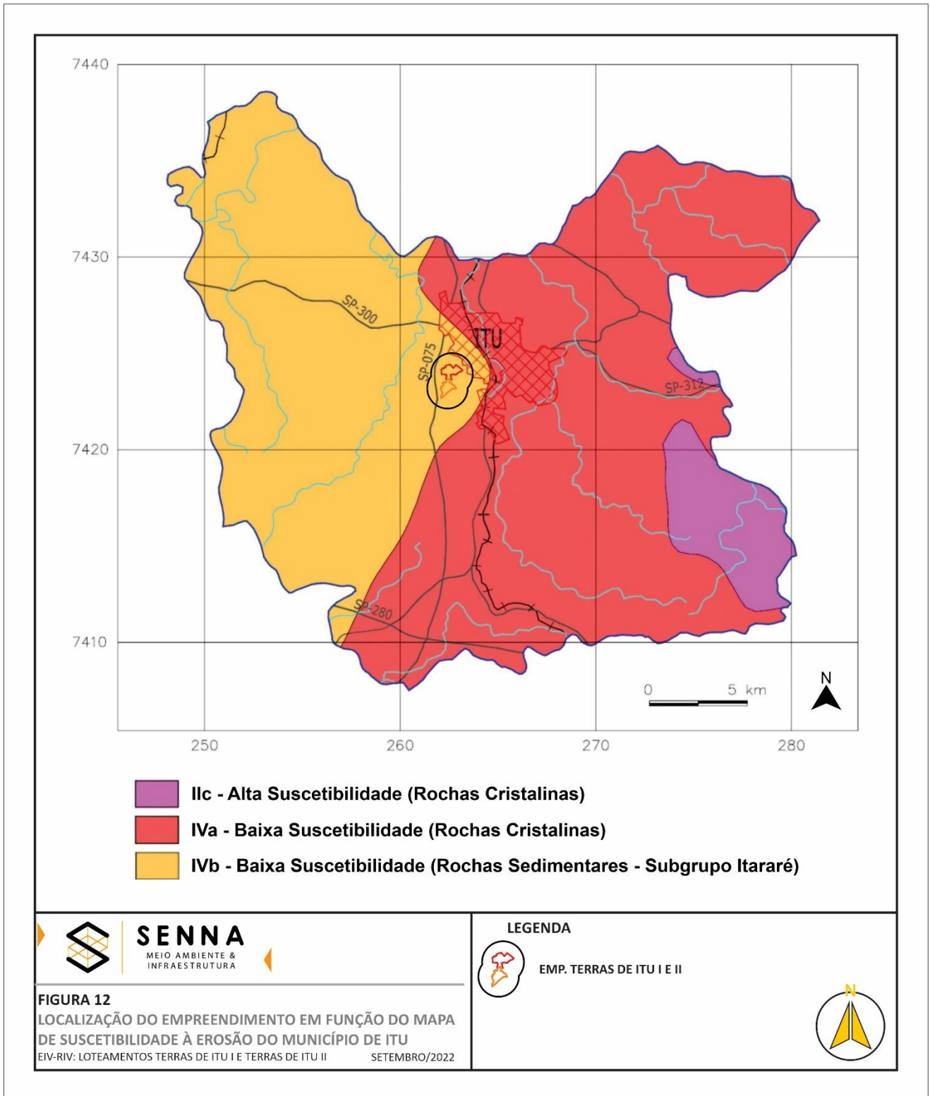
FIGURA 12: Localização da área, em função do Mapa de Suscetibilidade à Erosão do município de Itu (adaptado de IPT, 1997).
