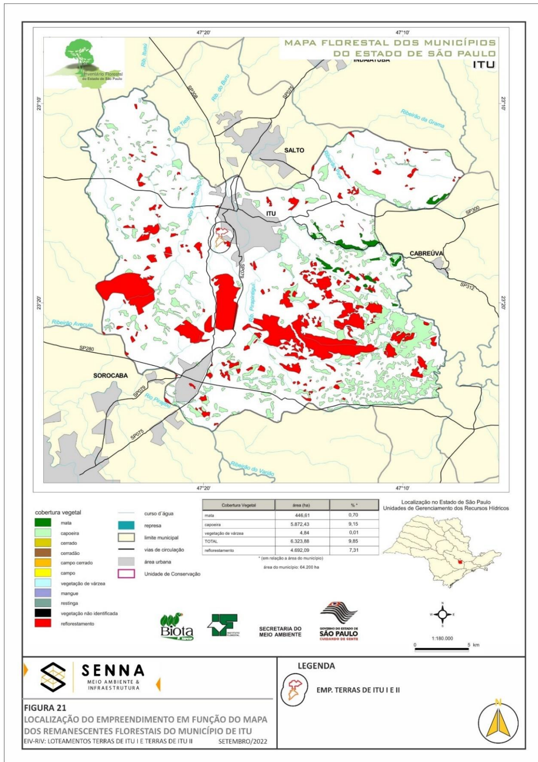
FIGURA 21: Localização da ADA (roxo) em função do mapa dos remanescentes florestais do município de Itu (Instituto Florestal do Estado de São Paulo).
