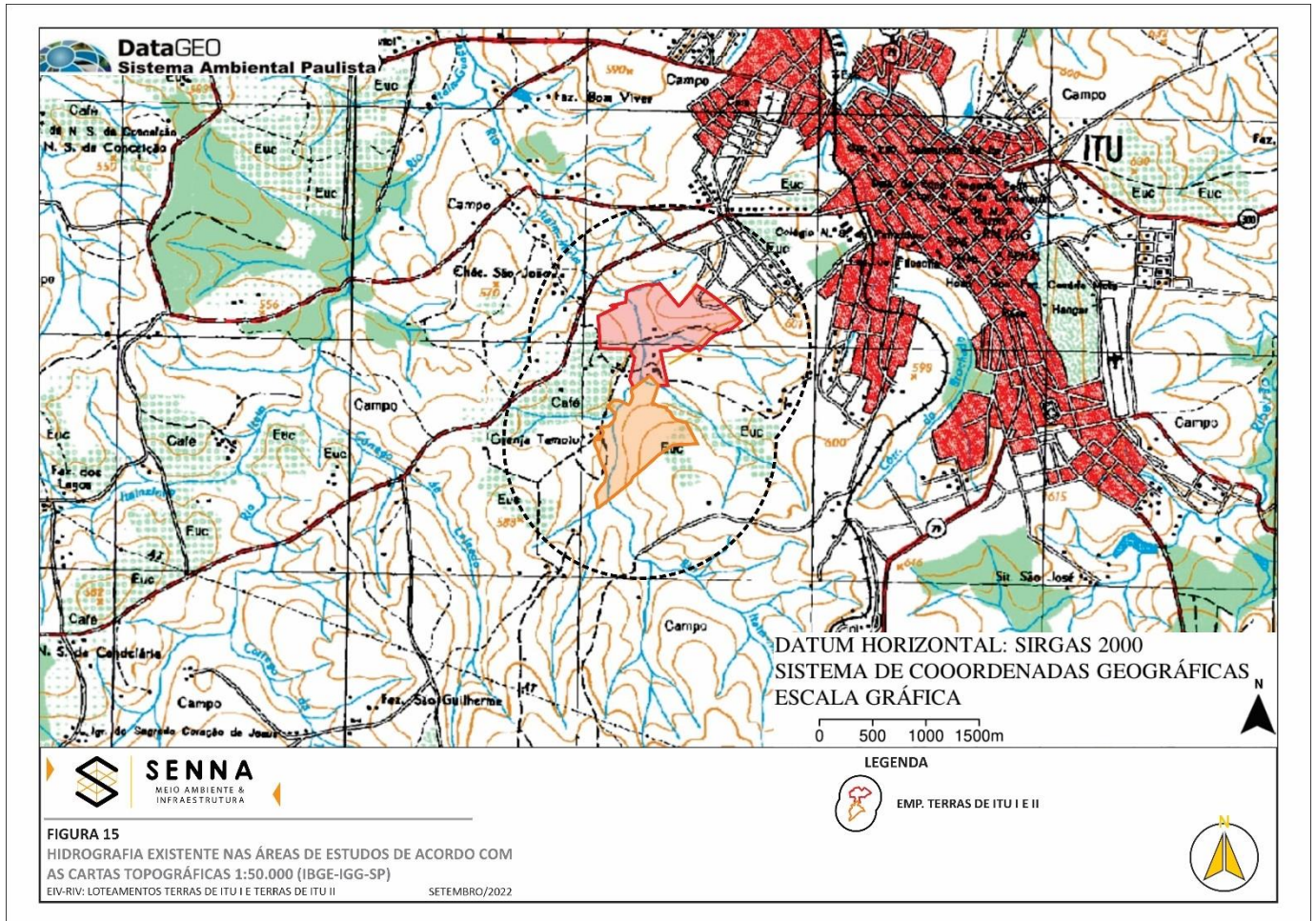
FIGURA 15: Localização da área de estudos em função da hidrografia existente na região.
