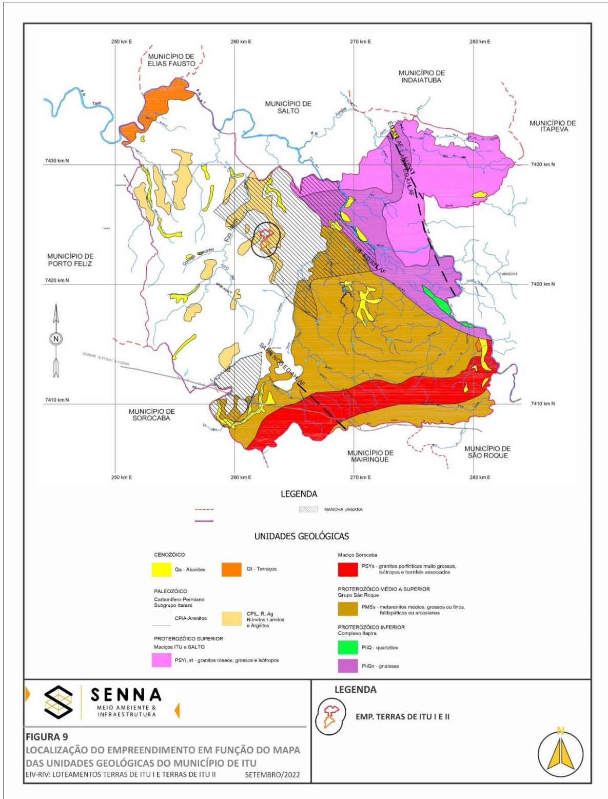
FIGURA 9: Localização da área, em função das unidades geológicas predominantes na região do município de Itu (adaptado de CPRM, 2010).
