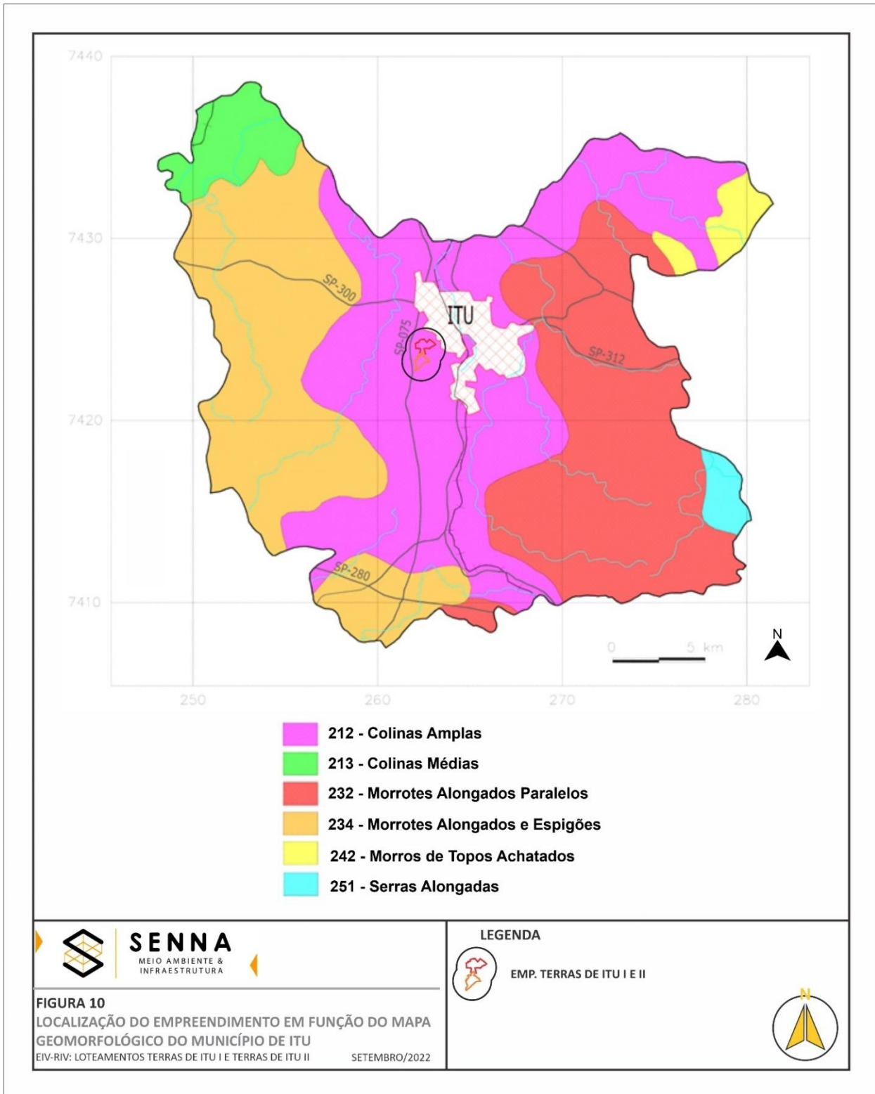
FIGURA 10: Localização da área, em função do Mapa Geomorfológico do município de Itu (adaptado de IPT, 1981).
