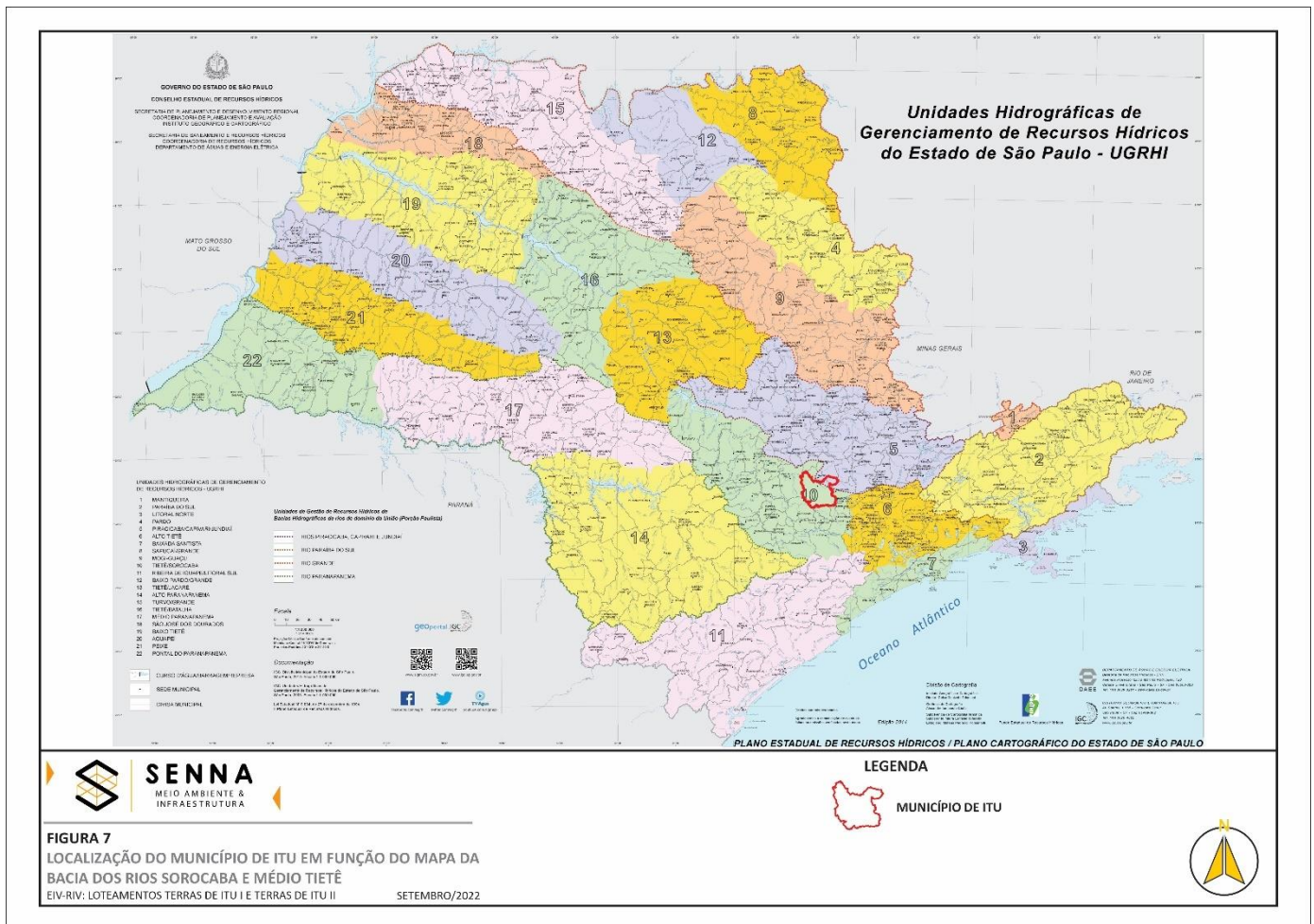
FIGURA 7: Localização do município de Itu, em função do Mapa da Bacia dos Rios Sorocaba e Médio Tietê.
