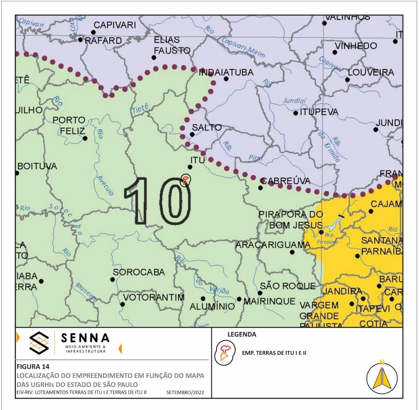
FIGURA 14: Localização da área de estudos, em função do mapa das UGRHs do Estado de São Paulo.
