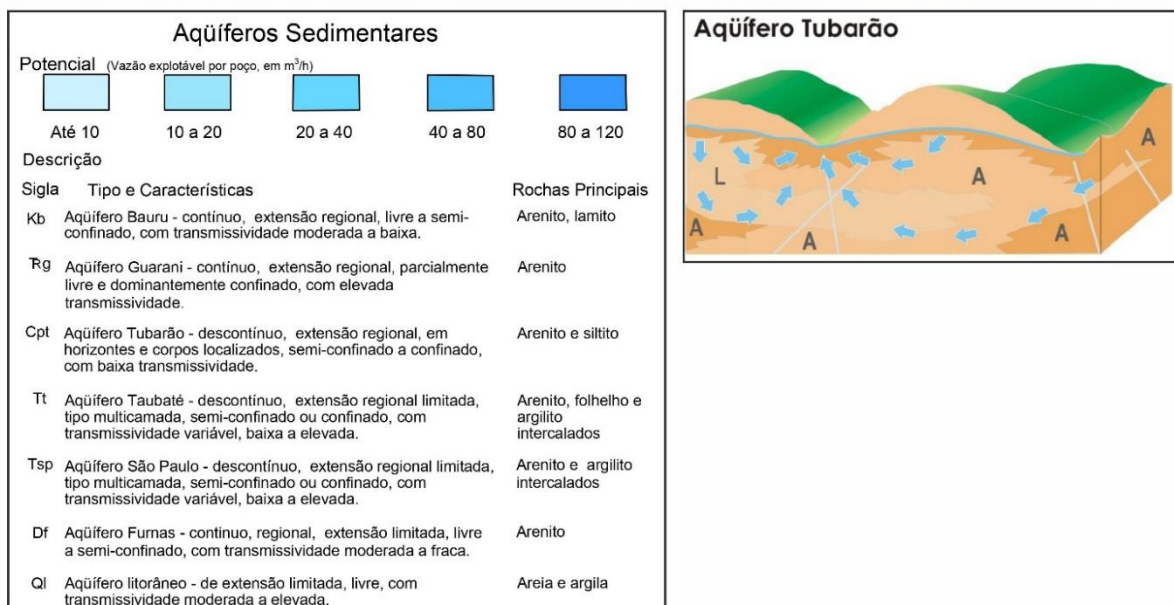
FIGURA 13: Localização da área de estudos, em função de sua hidrogeologia, conforme Mapa de Águas Subterrâneas do Estado de São Paulo.
