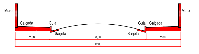
CORTE TRANSVERSAL DAS RUAS 01,02,04,08,09,14,15,16 E 18 ESCALA:- 1:100
