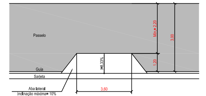
DETALHE DE RAMPA DE ACESSO ESCALA:- 1:100
