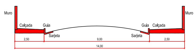
CORTE TRANSVERSAL DAS RUAS 03,05,06,07,10,11,12,13,17,19,20 E 21 ESCALA:- 1:100
