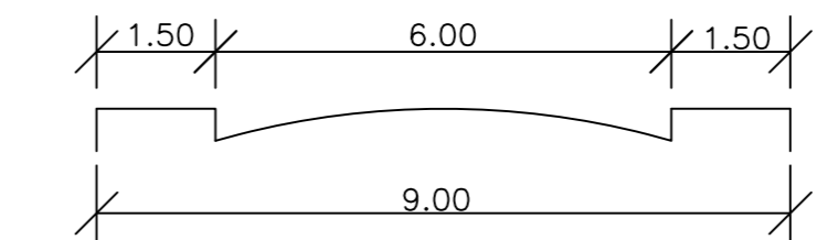
PERFIL TRANSVERSAL RUA 'A'
