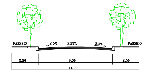
PERFIL TRANSVERSAL DAS RUAS ESCALA 1:200
